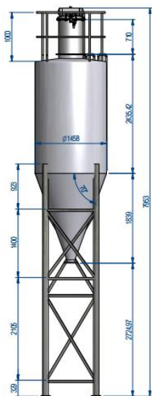
4 m3 Silo
