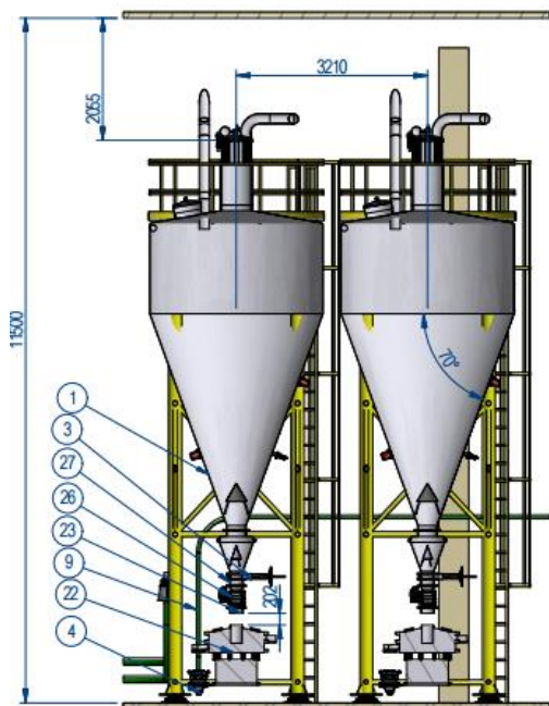
20 m3 Silo
