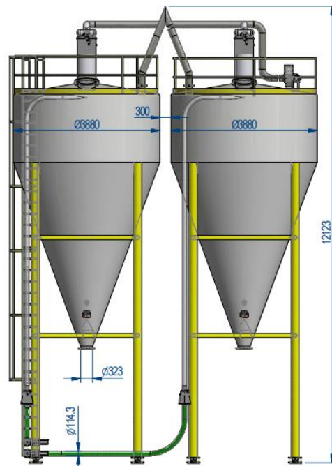
30 m3 Silo
