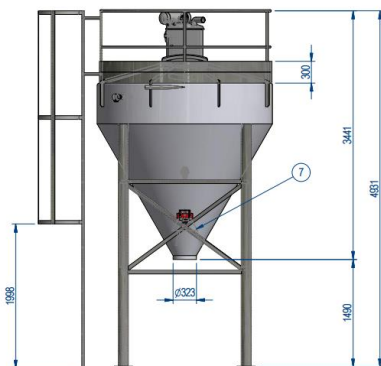
6 m3 Silo
