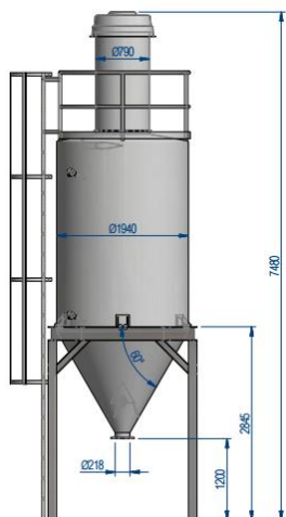
4 m3 Silo
